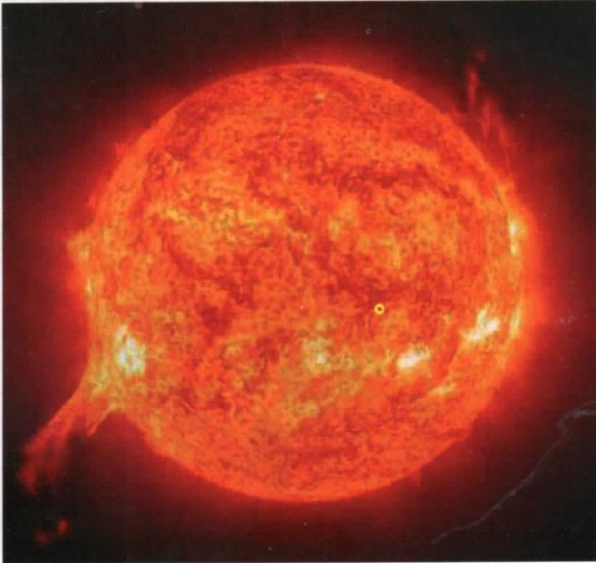
نتوء ضخم رصدته المركبة (سوهو) فى عام ٢٠٠٢. انظر [الكروموسفير والهالة والرياح الشمسية]
