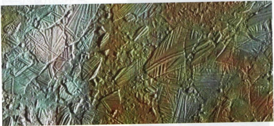
السطح المُكوّن من التلوج المُهشّمة للقمر (أوروبا) التابع لكوكب المُشترى. وترجع اختلافات الألوان إلى ترسّبات الجسيمات الدقيقة من التلوج. والصورة مركبة من مجموعة من الصور التقطت خلال عمليات رصد قامت بها المركبة (جاليليو) بين عامي ١٩٩٦ و ١٩٩٧. انظر [أقمار المُشترى]
