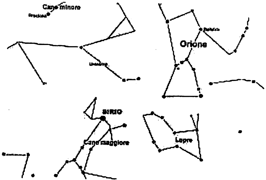
شكل (٢٠) الشعرى والجبار في السماء تصميم المؤلف
