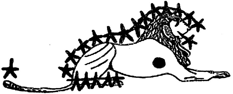
شكل (٢٦) كوكبة الأسد (سقف حجرة دفن سبتي الأول) تصميم لورنزو مارجاكى
