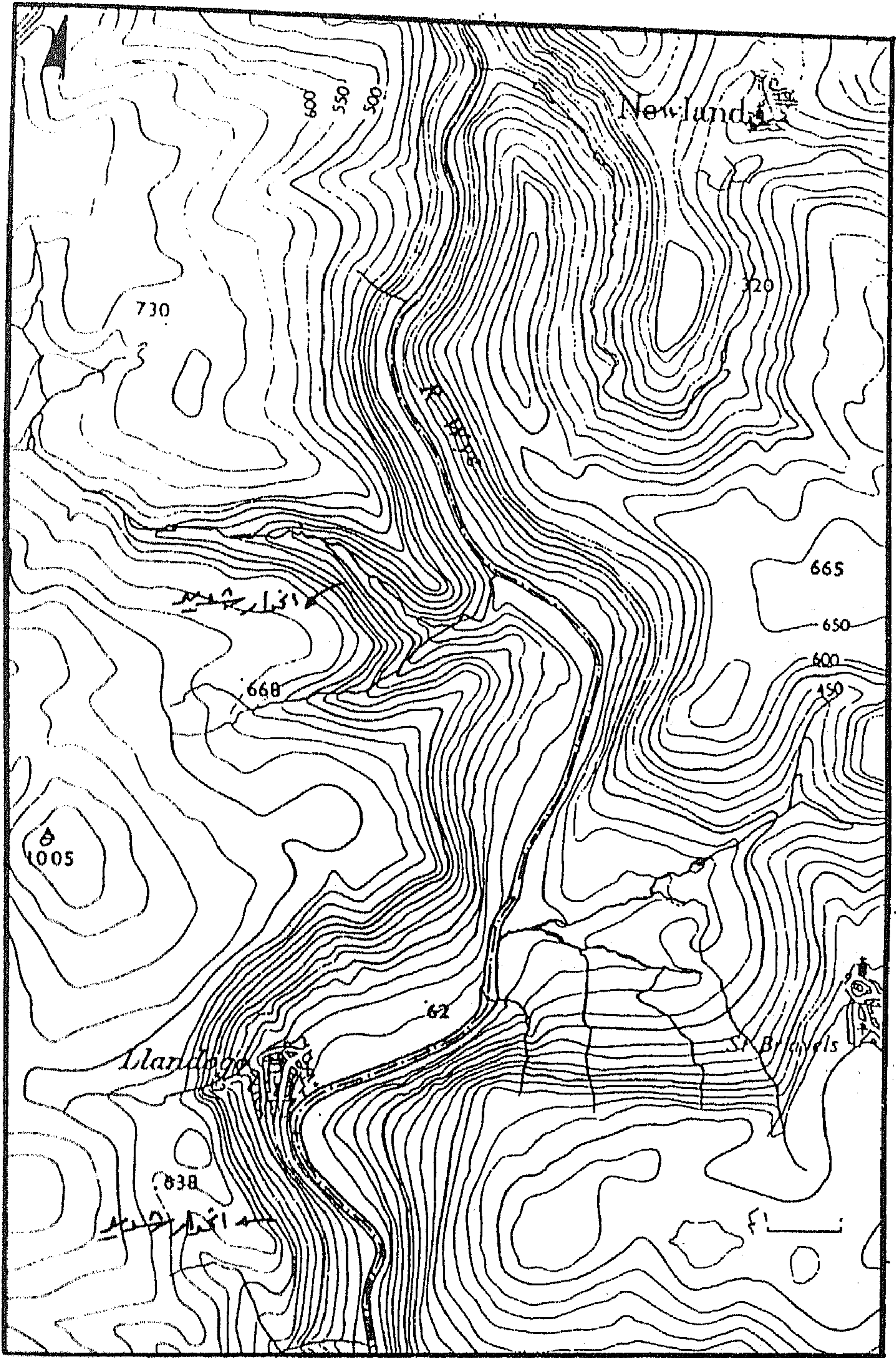
شكل رقم (١٢) تمثيل ظاهرة الحافات الرأسية والجروف
