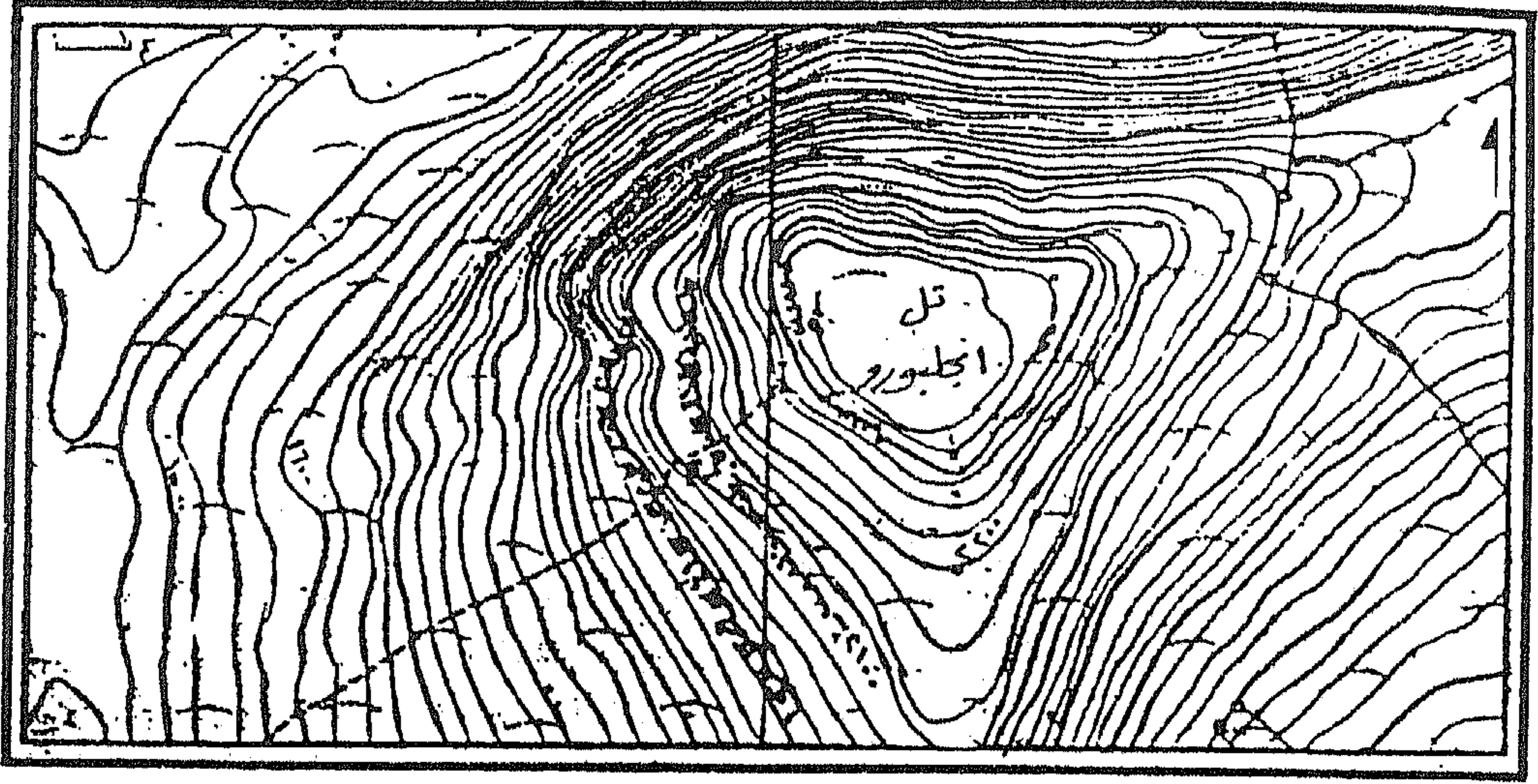
شكل رقم (۳۰) سفوح شديدة الانحدار بجبال بنين
