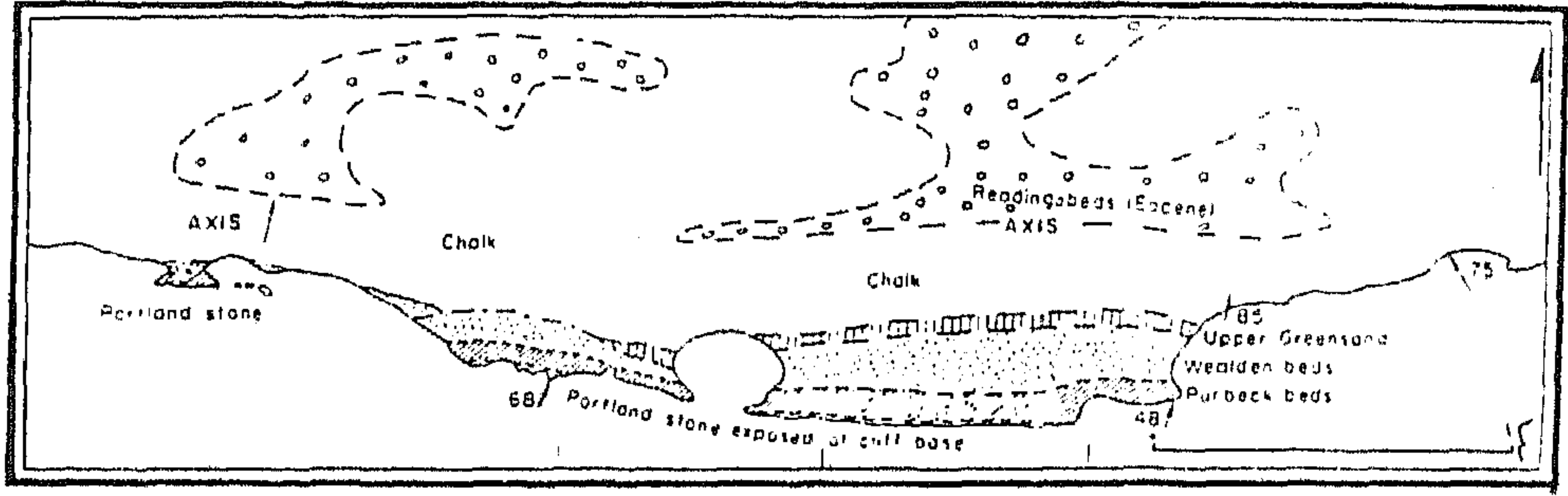
شكل رقم (١٠٥) الخريطة الجيولوجية لساحل دورست (منطقة كهف لولوورث)
