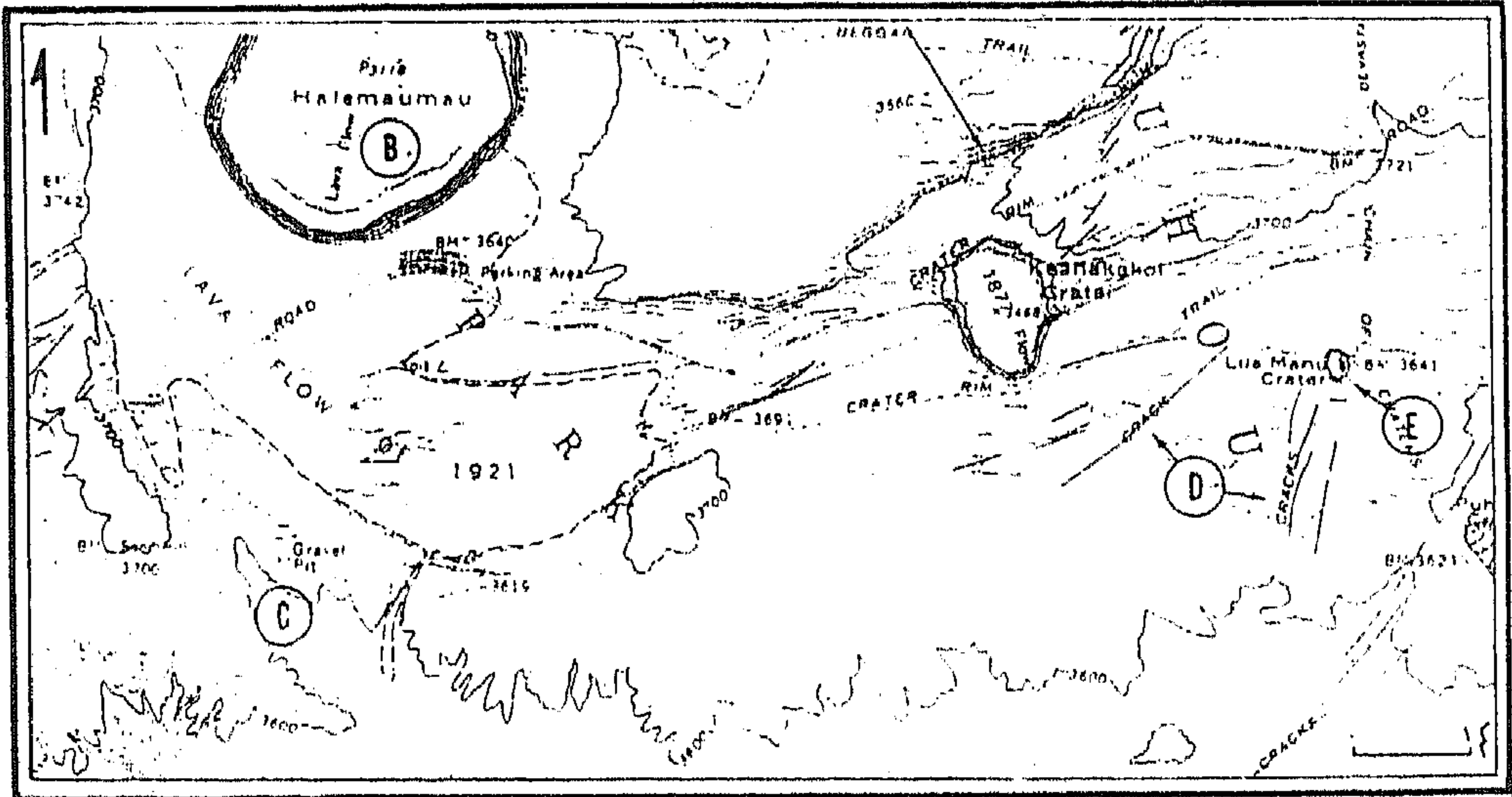
شكل رقم (٥١) فوهة بركان كىلاواى على السفوح الجنوبية الشرقية بقبو بركان مونالوا
