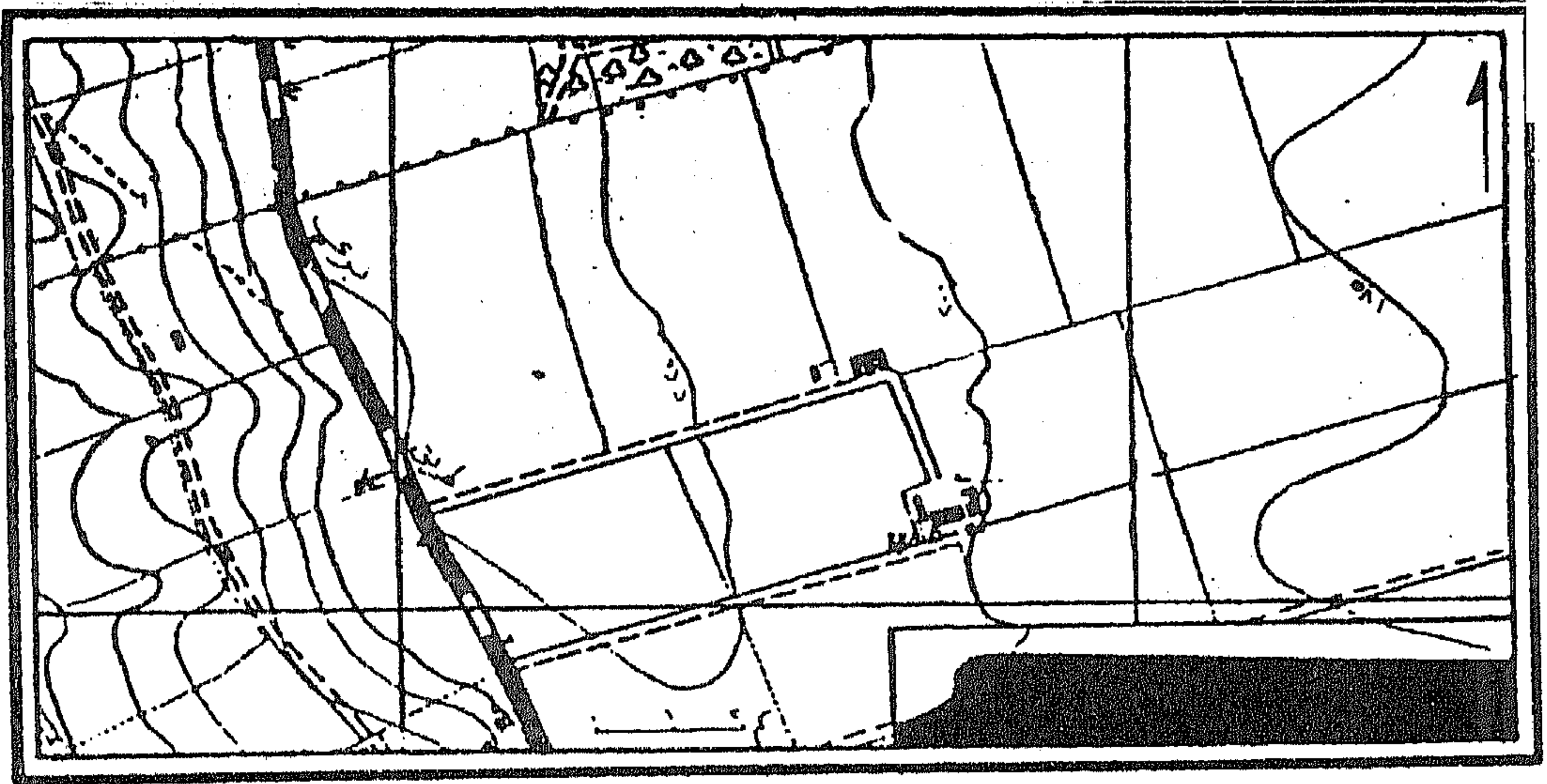
شكل رقم (٣٢) كويستا (حافة وانحدار ميل)
