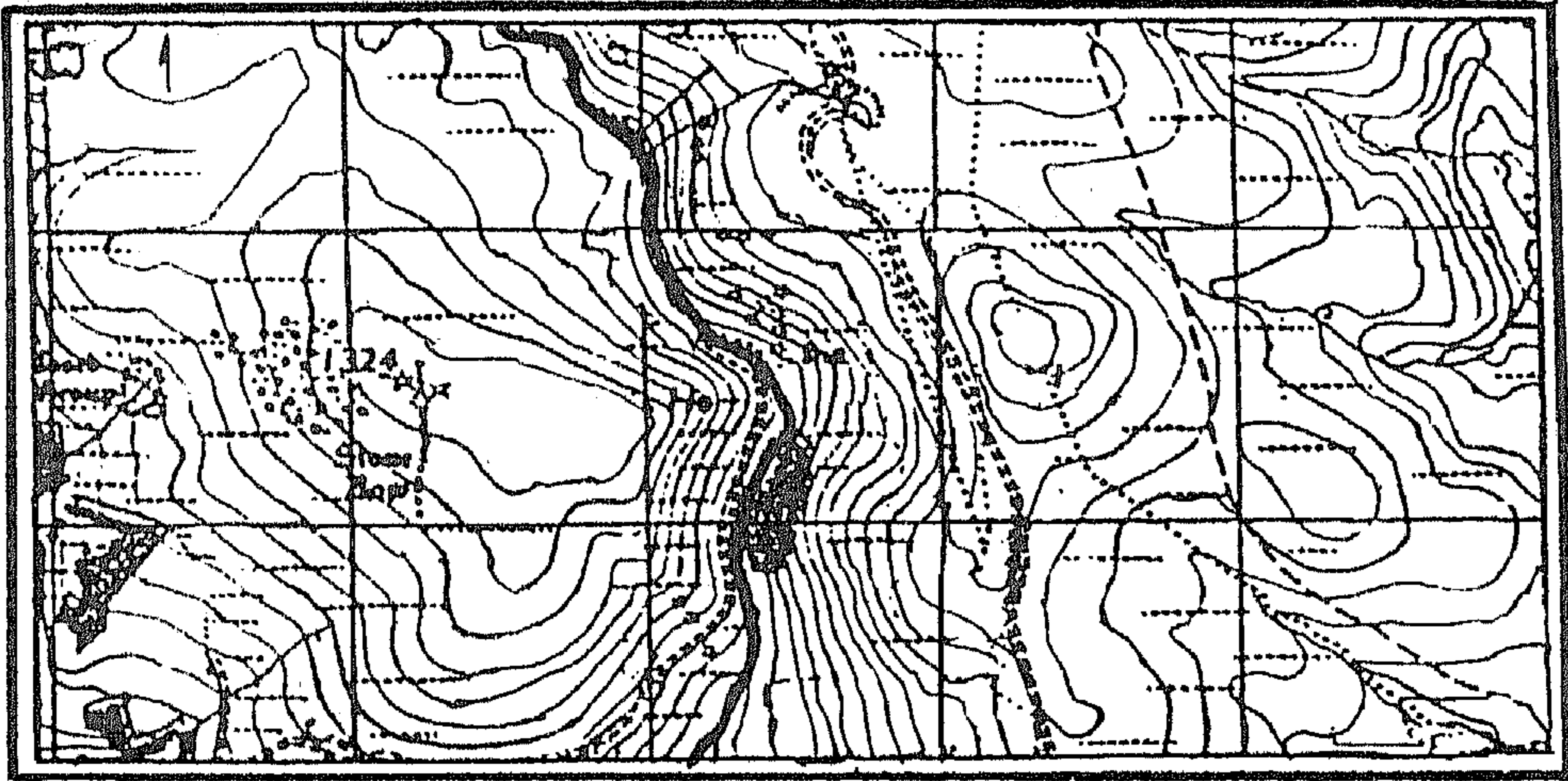
شكل رقم (٣٧) وادي ضيق ذو جوانب شديدة الانحدار
