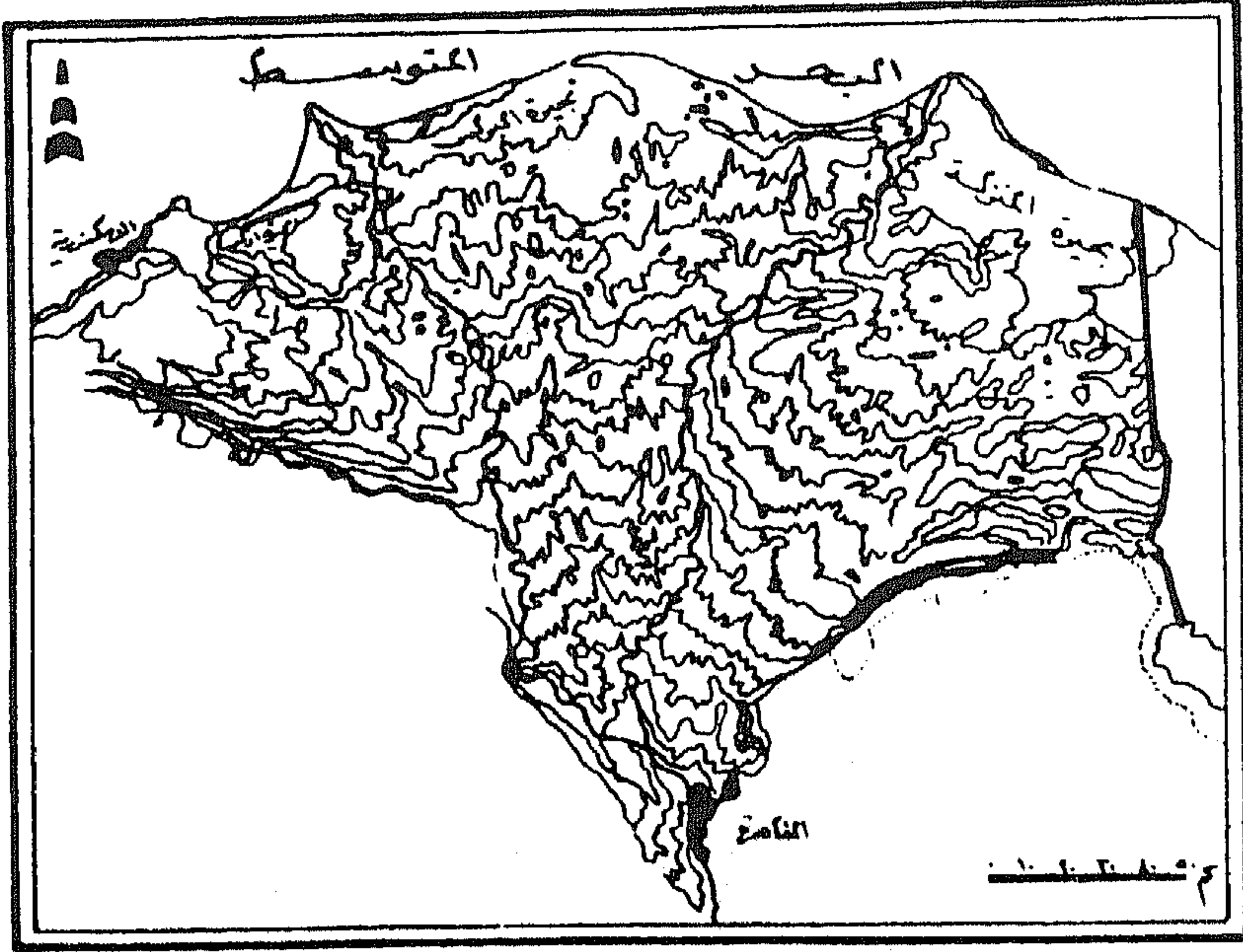
شكل رقم (٧٨) الخريطة الكنتورية لدلتا نهر النيل
