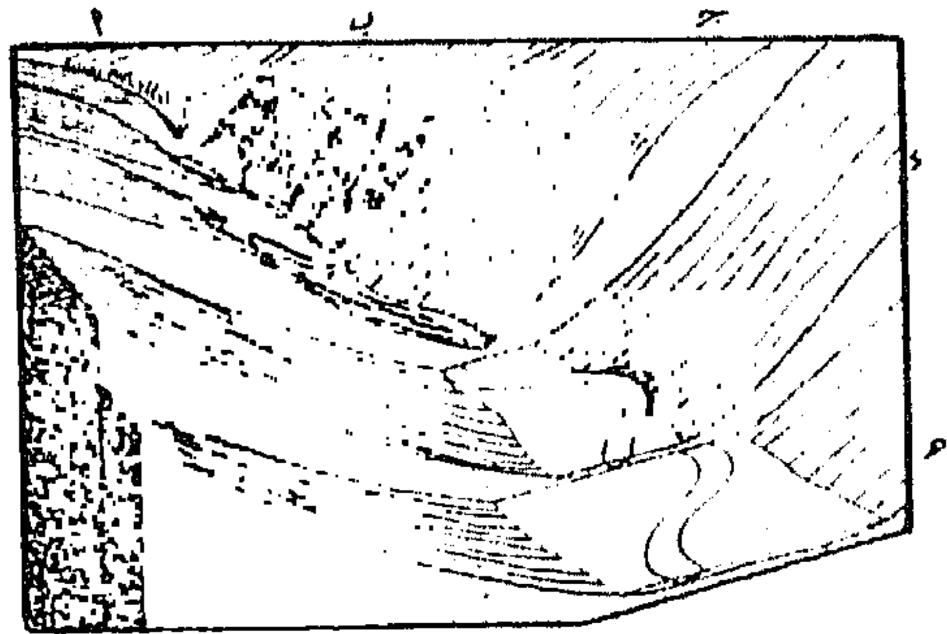
شكل رقم (١٤٠) مراحل الأودية النهرية
