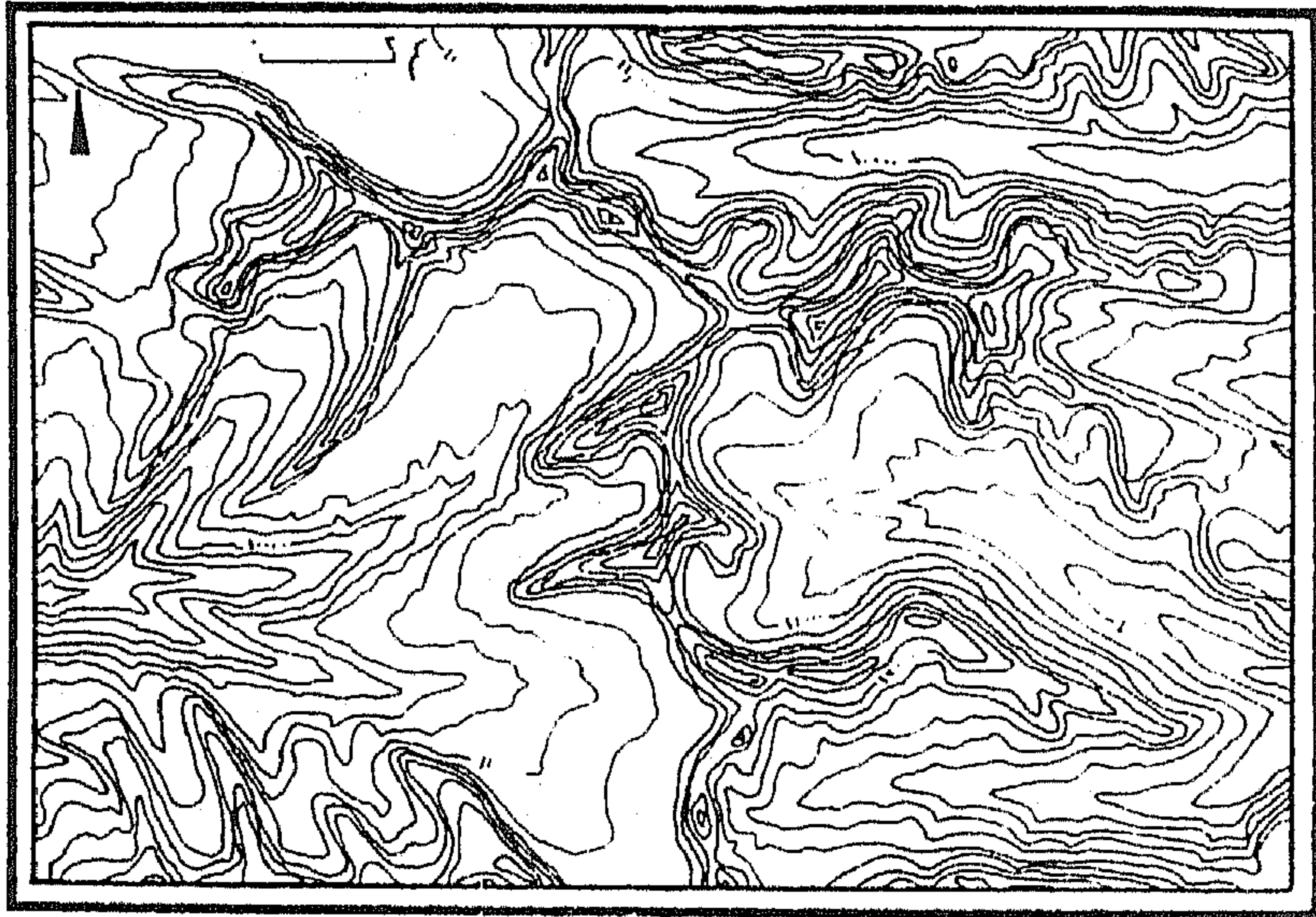
شكل رقم (١٢٠) جزء من سلسلة جبال يوثينا الكبرى فى ولاية يوتا تسودها التعرية الجبلية
