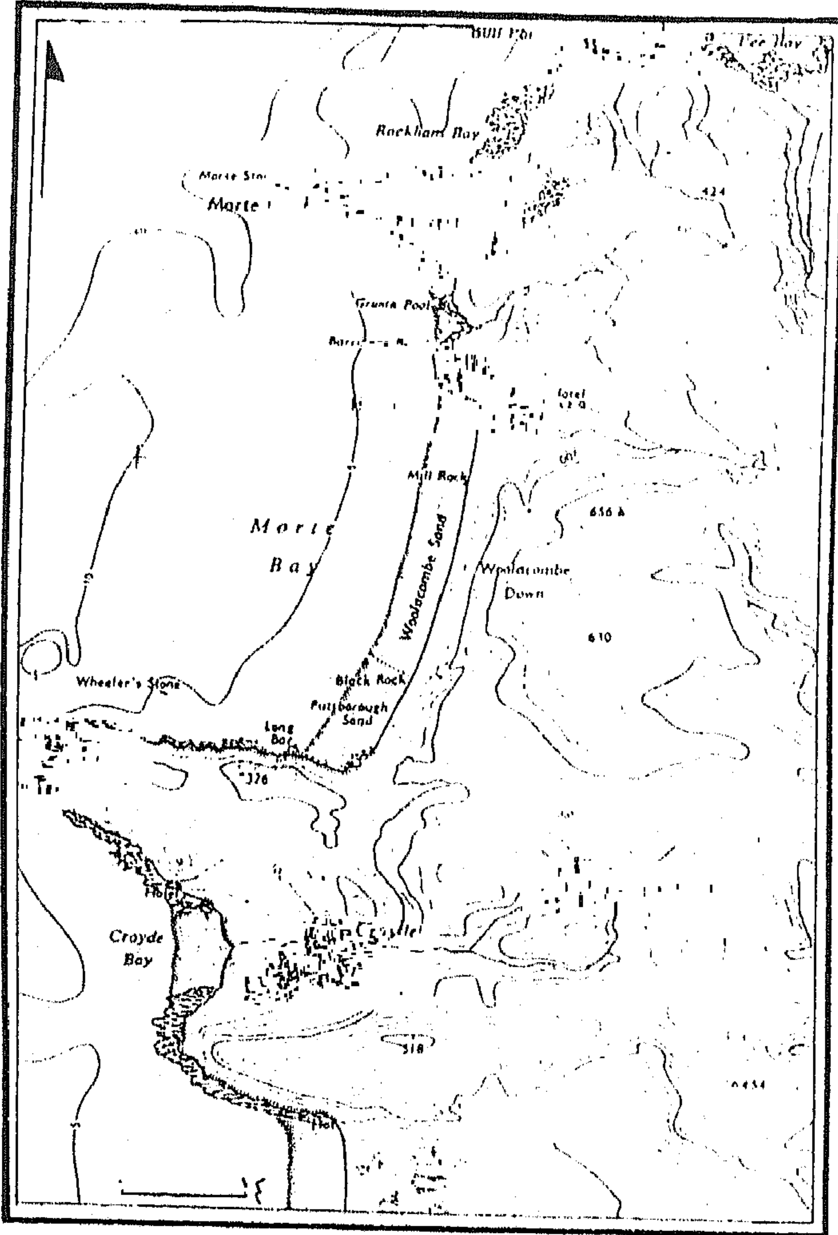
شكل رقم (١٠٣) جزء من ساحل ديهلون (خليج وولاكومب)
