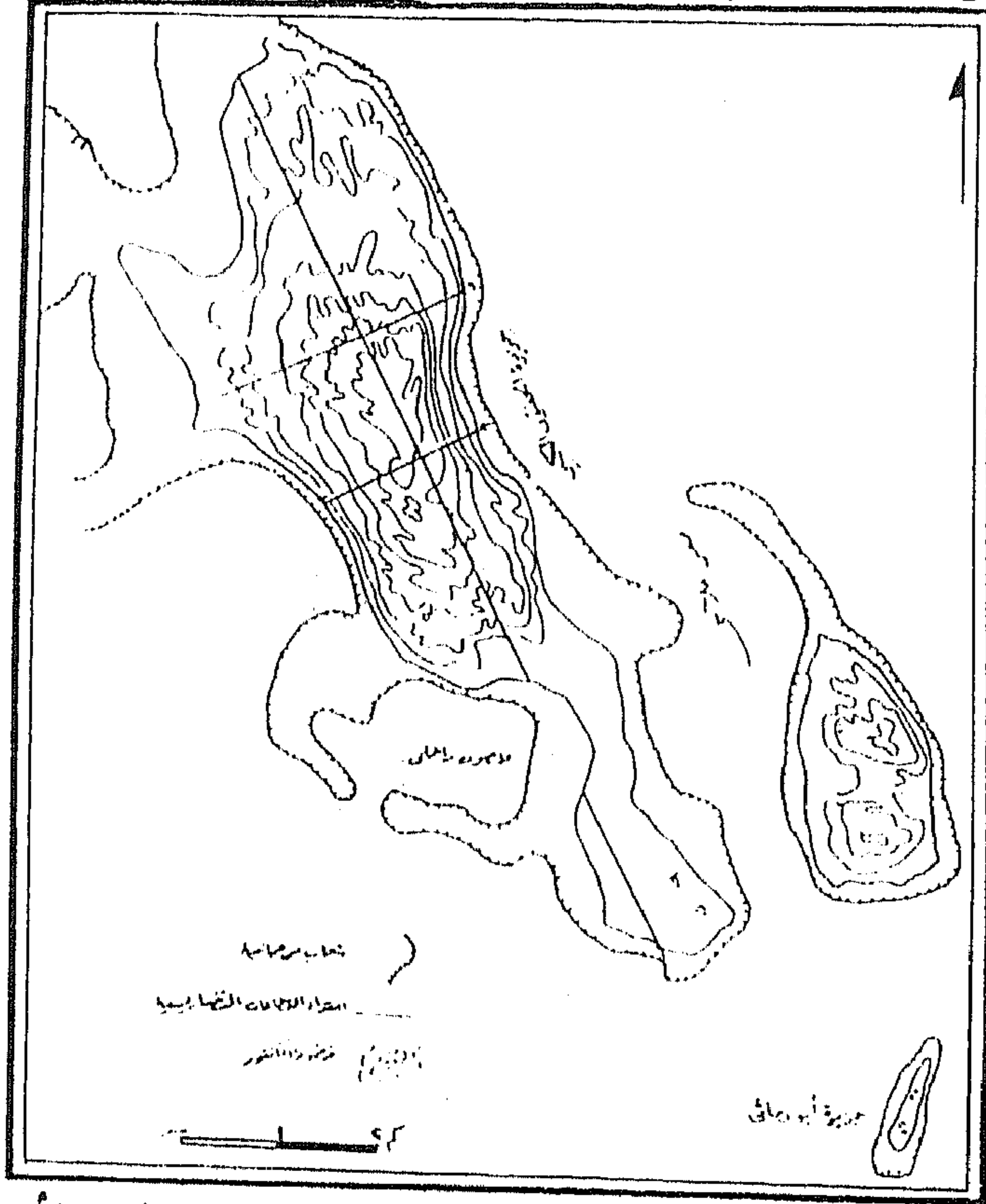
شكل رقم (١١٤) جزيرتا الجفتون الكبير والجفتون الصغير بالبحر الأحمر
