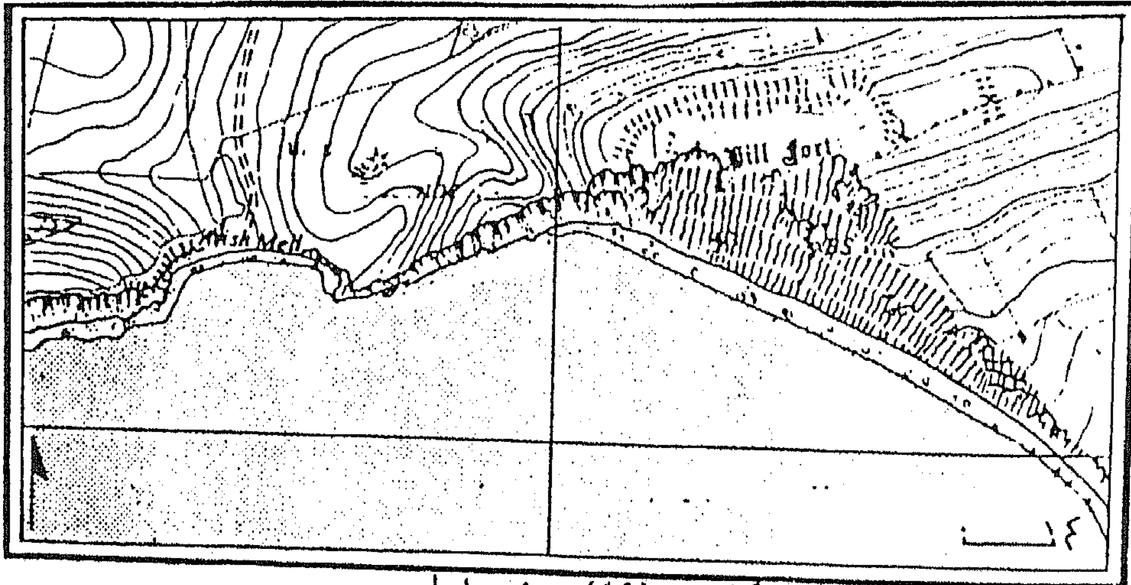
شكل رقم (٤٩) جرف ساحلي
