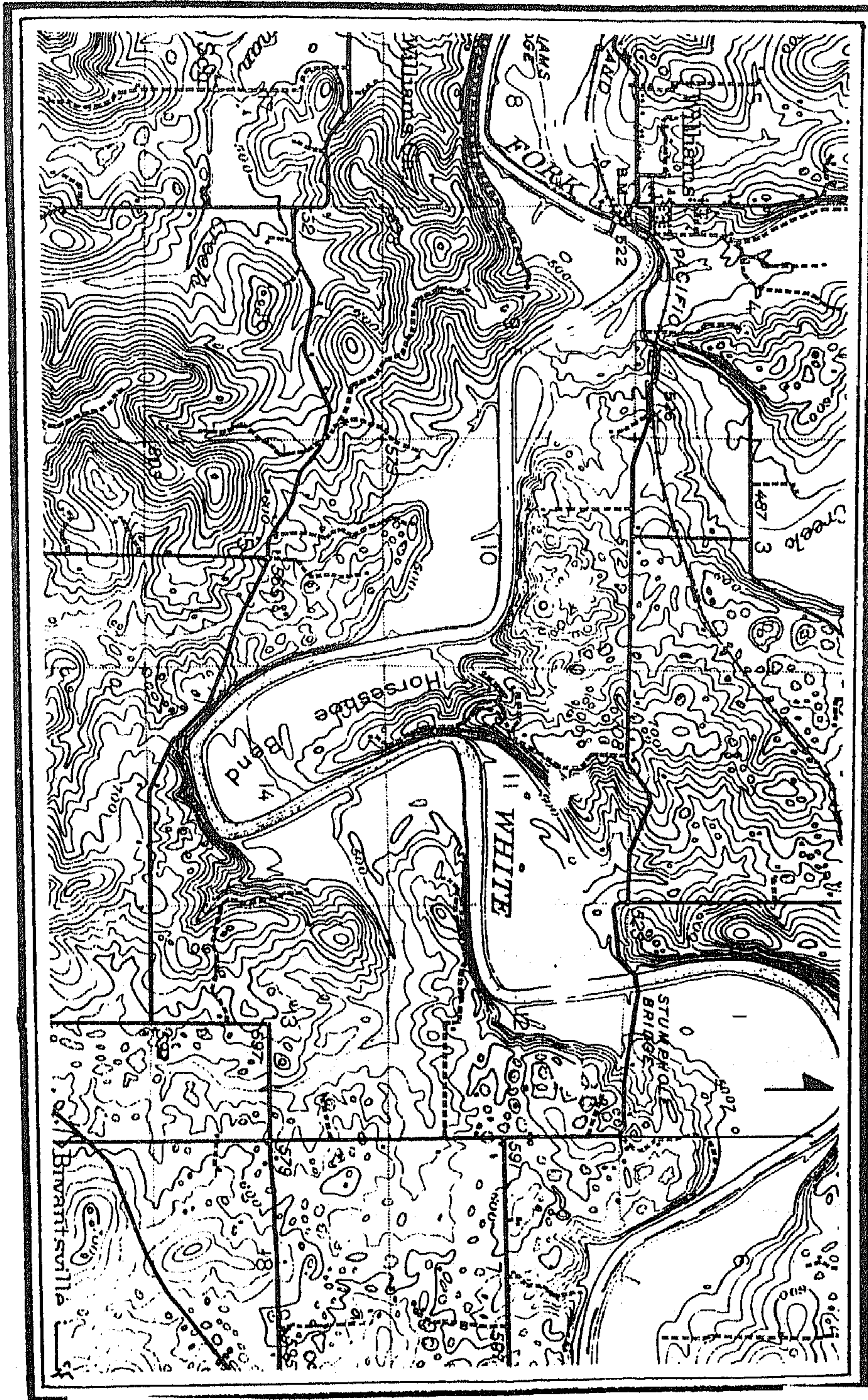
هككل رقم (٧٣) جزء من نهر هوايت بولاية أندياتا الأمريكية
