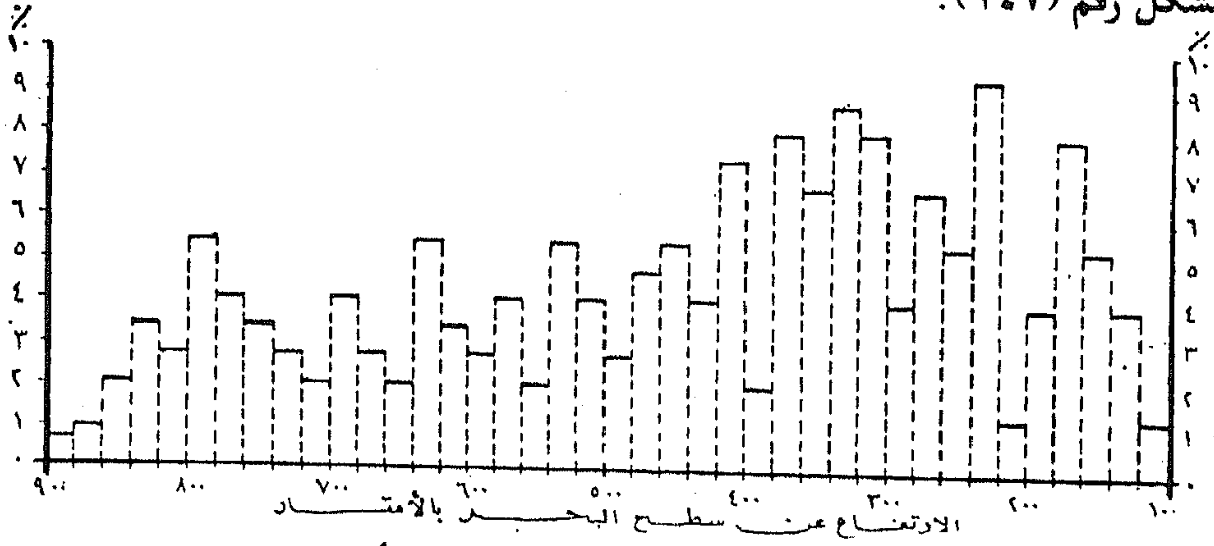
شكل رقم (١٤٧) طريقة إنشاء المنحنى الألتيمترى
