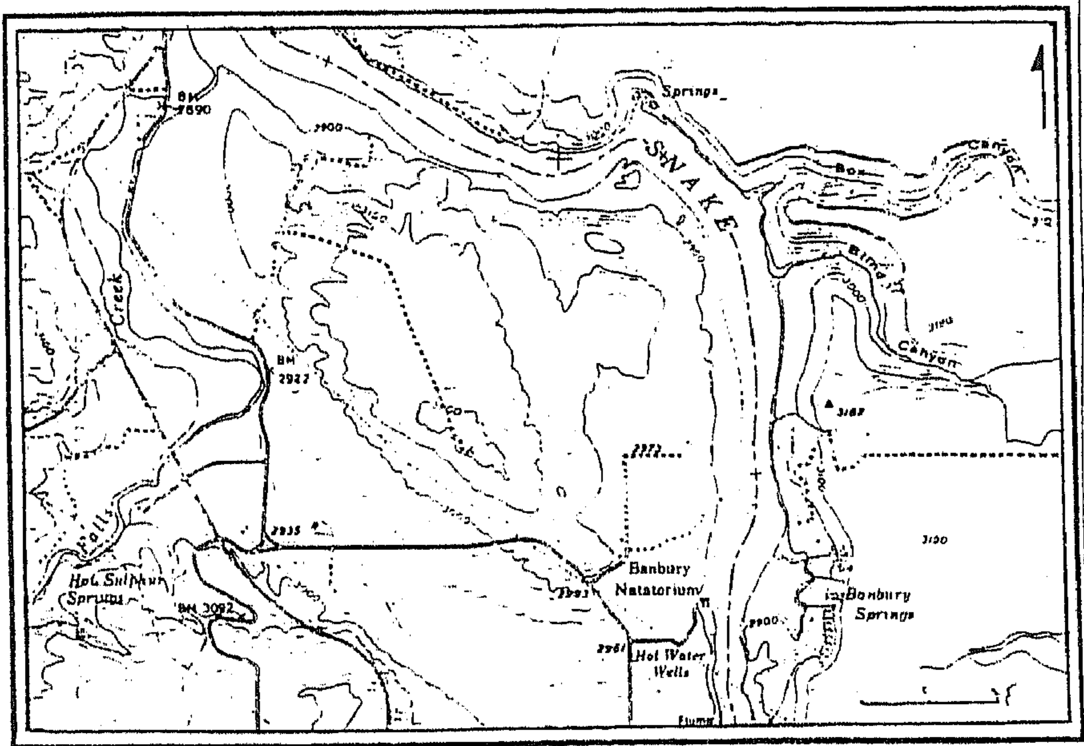
شكل رقم (٧٠) قطاع محدود من وادي سينيك بولاية إيداهو الأمريكية
