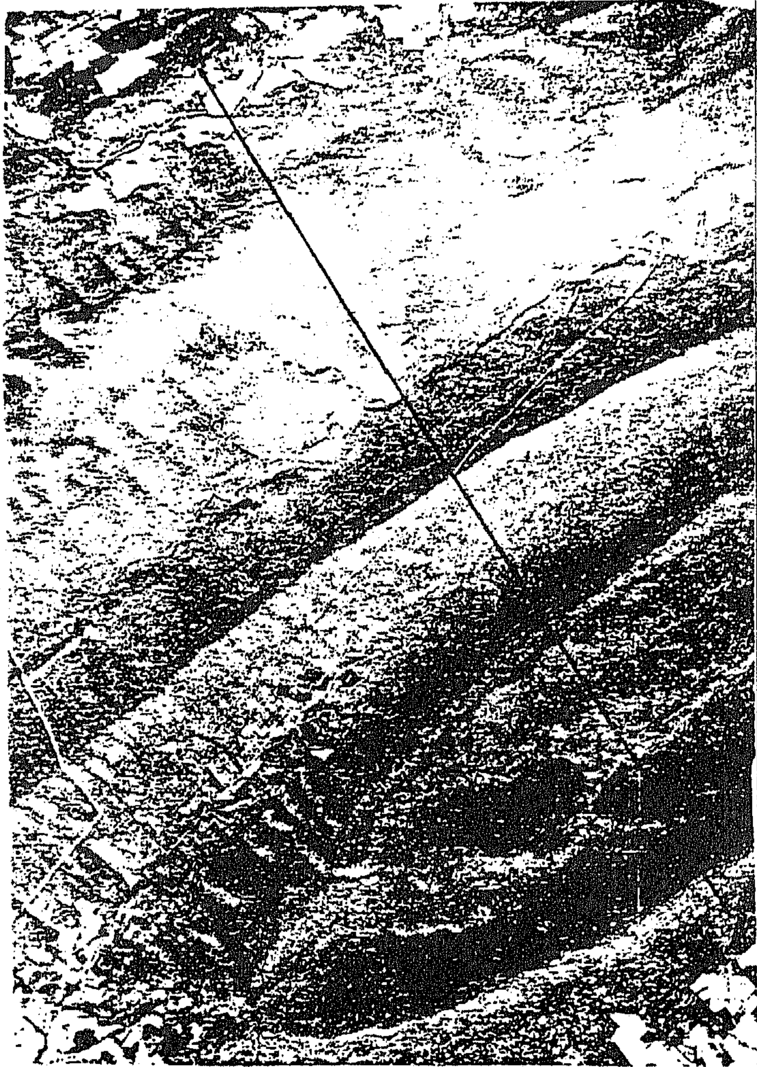
شكل رقم (٦٠) صورة جوية لحافات الأودية بجبال الأبلاتش.
