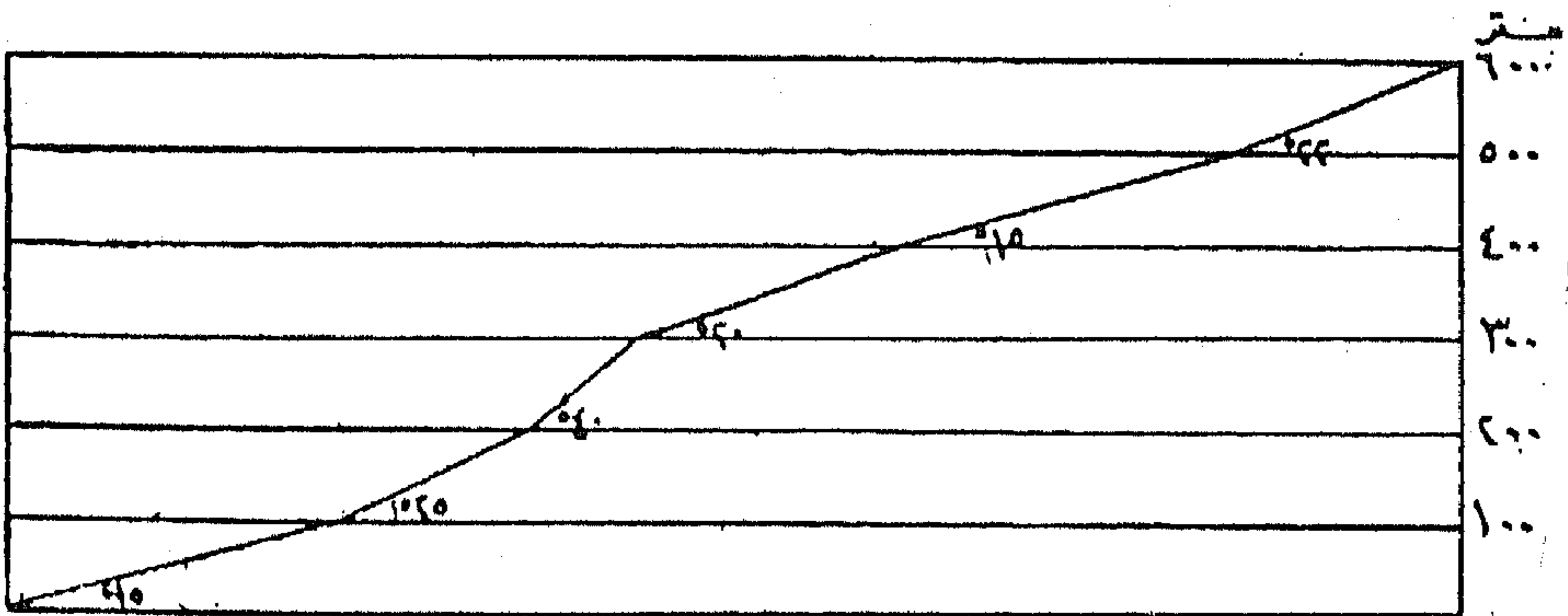
شكل رقم (١٤٦) المنحنى الكليينوجرافى
