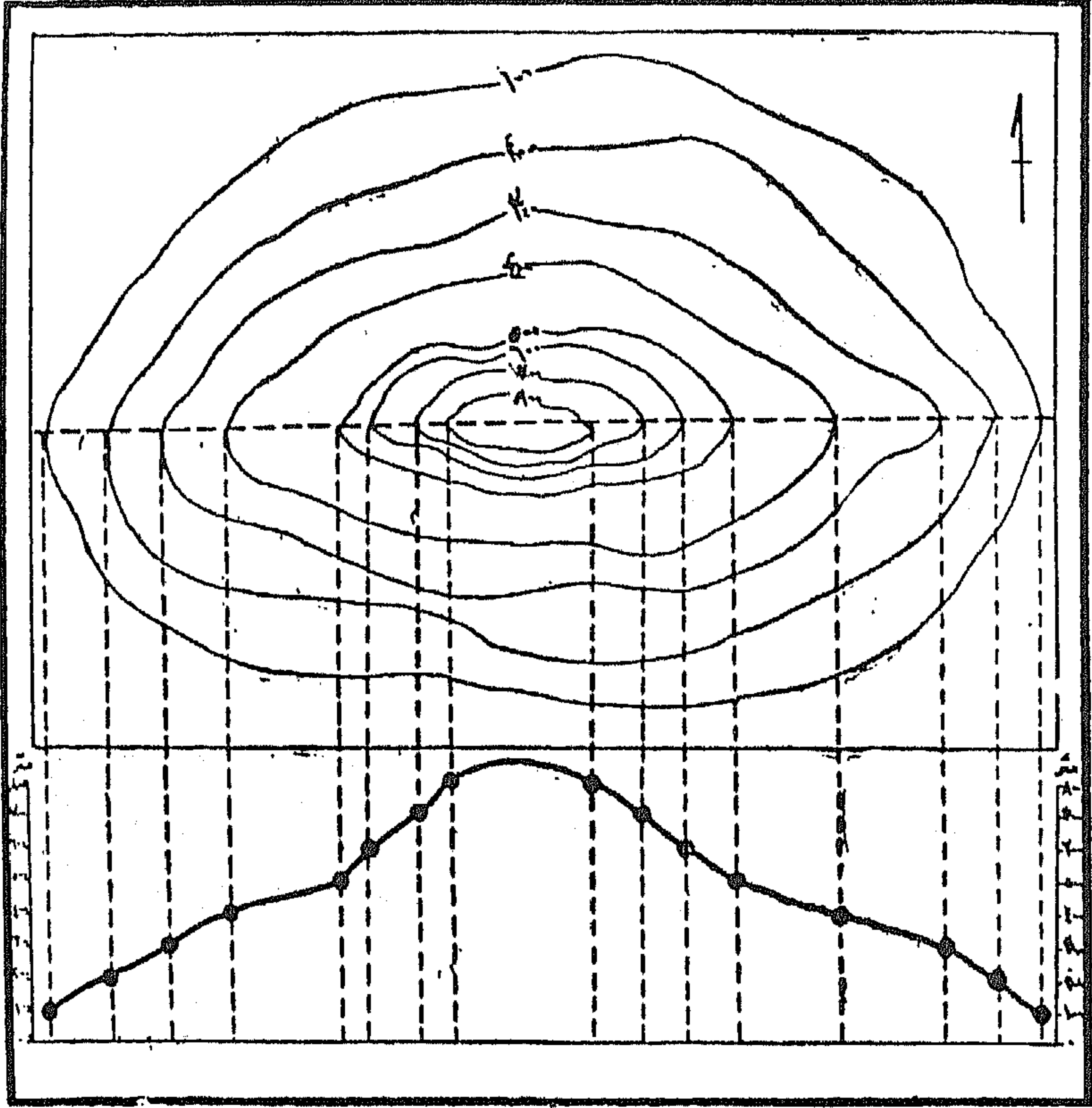
شكل رقم (١٣١) توقيت الأعمدة الرأسية اللازمة لرسم القطاع التضاريسي
