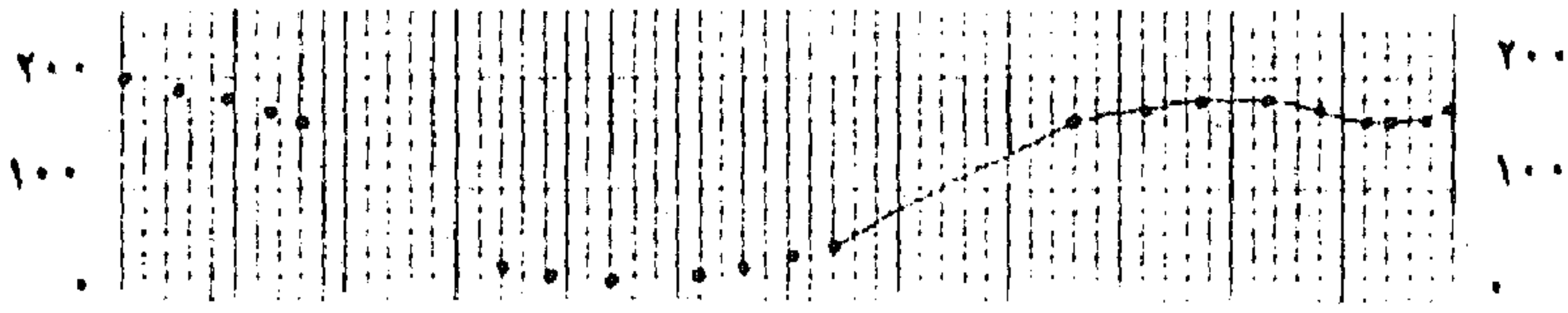
قطاع من الشمال إلى الجنوب
