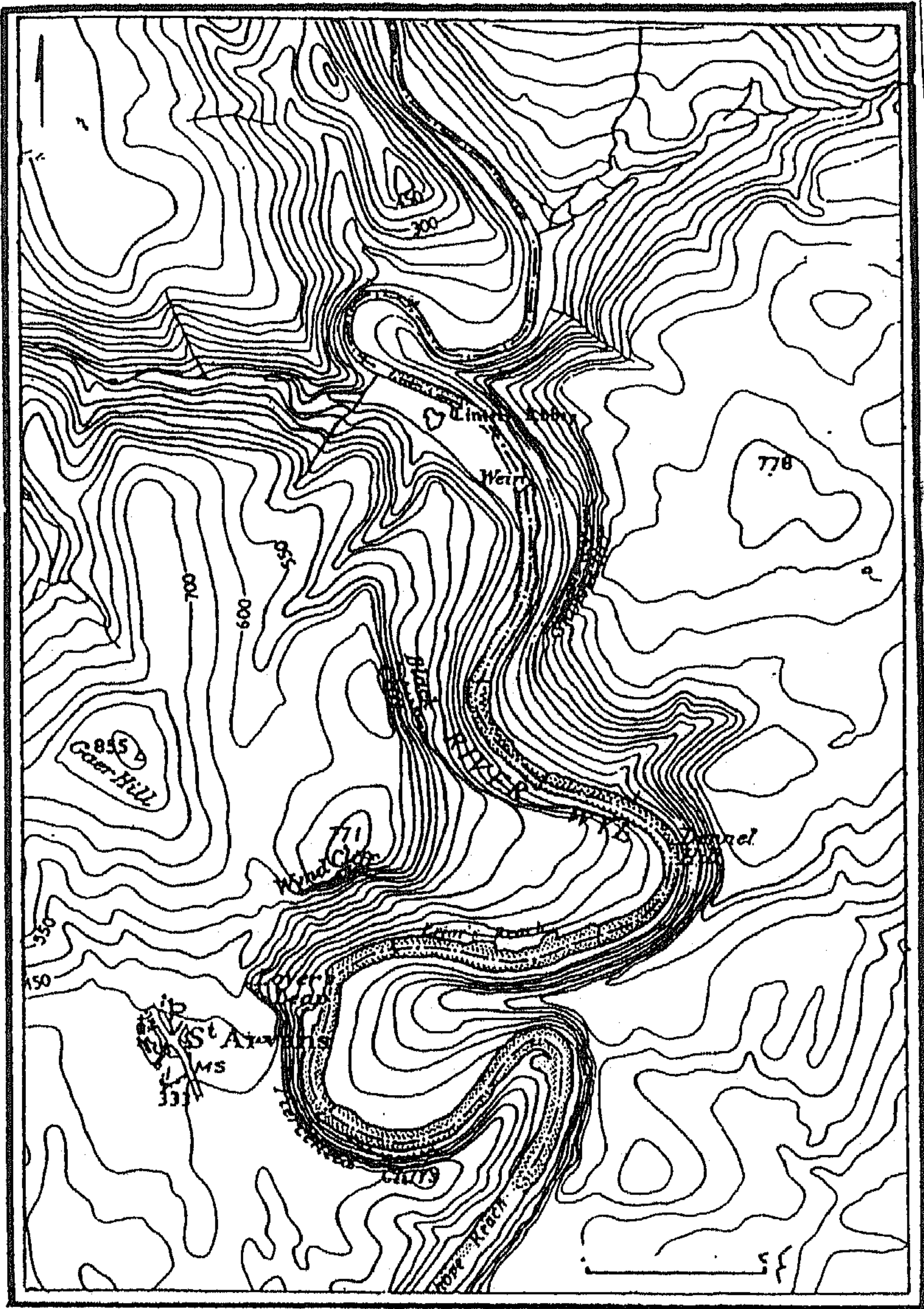
شكل رقم (٨١) الشياخات بقطاع في نهر واي بانجلترا
