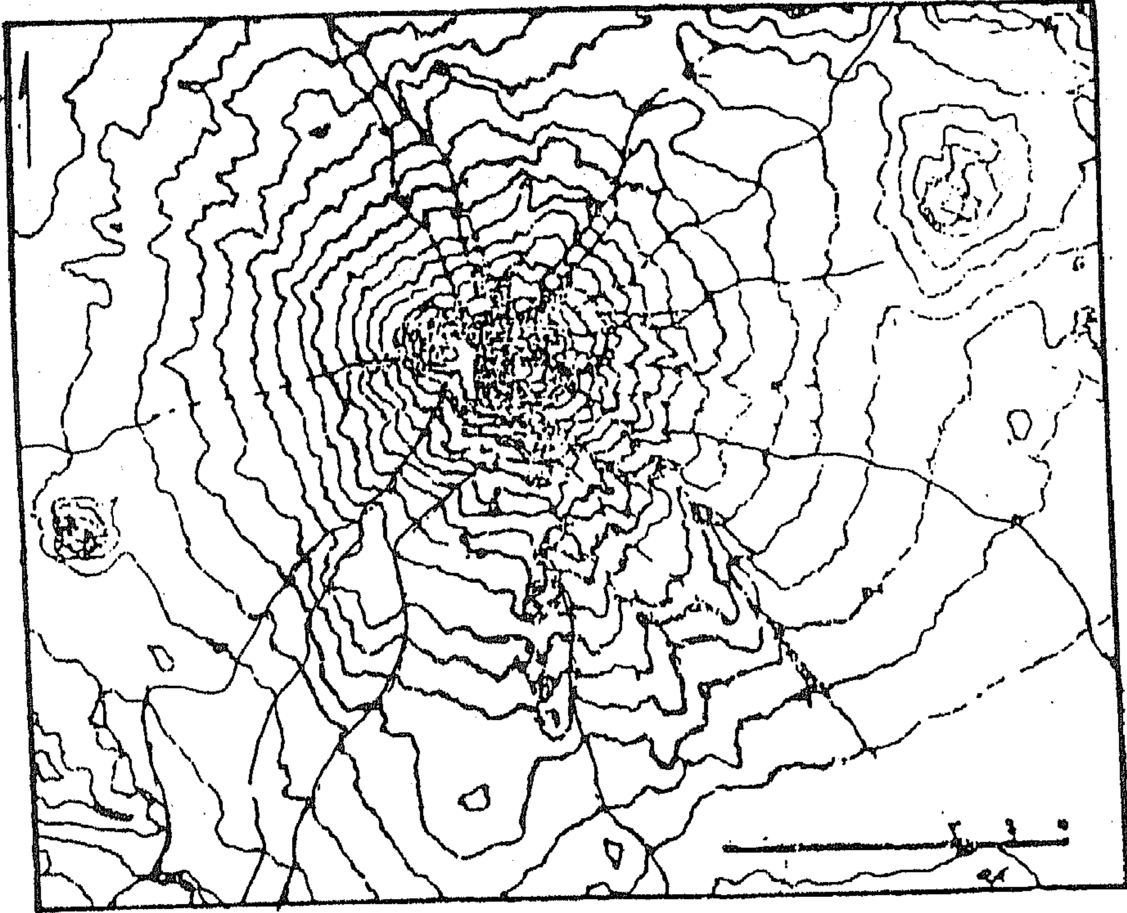
شكل رقم (٥٠) جبل شاستا المخروطي في سلسلة جبال كسكيد
