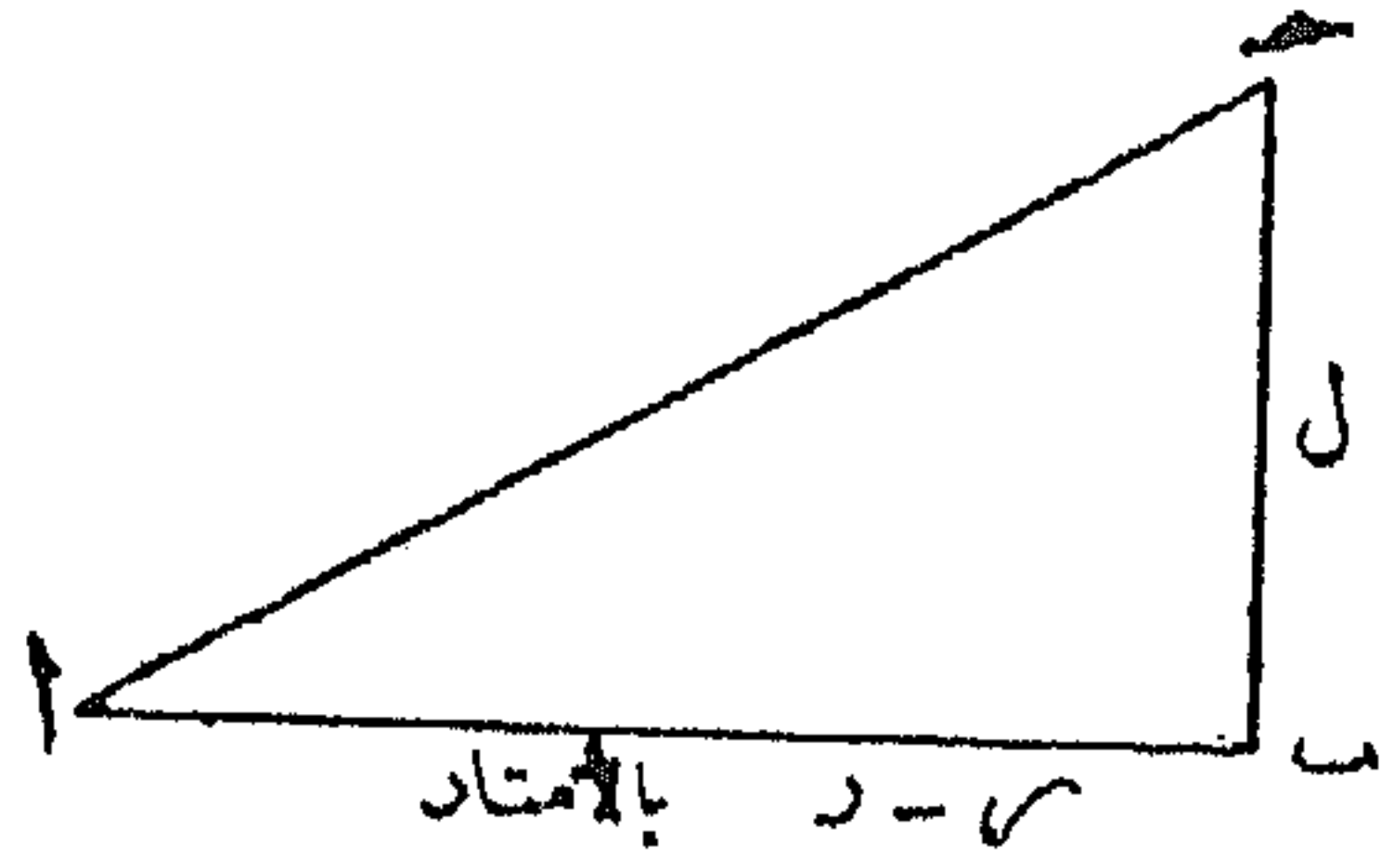
شكل رقم (١٤٥) فكرة المنحنى الكليينوجرافى
