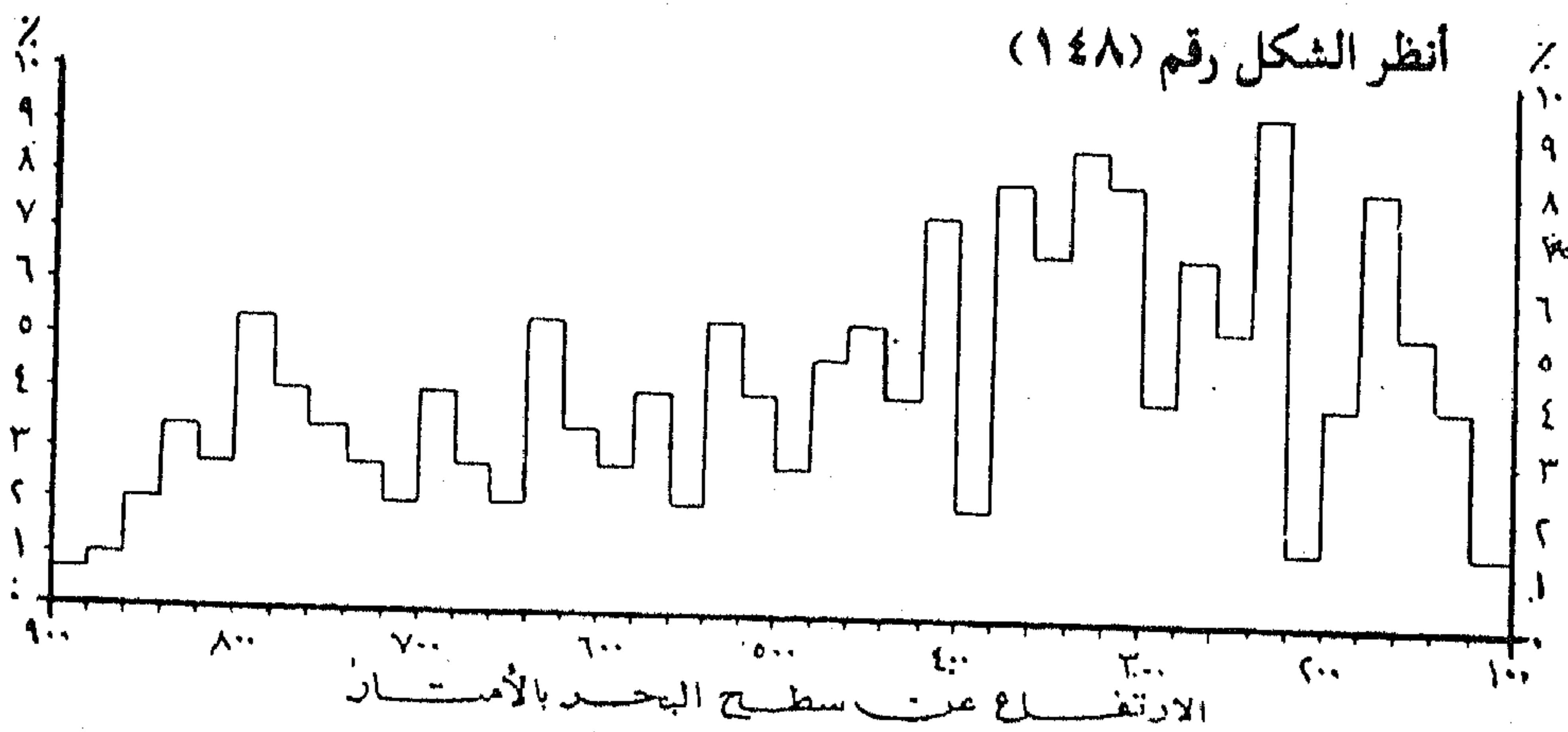
شكل رقم (١٤٨) المنحنى الألتيمترى
