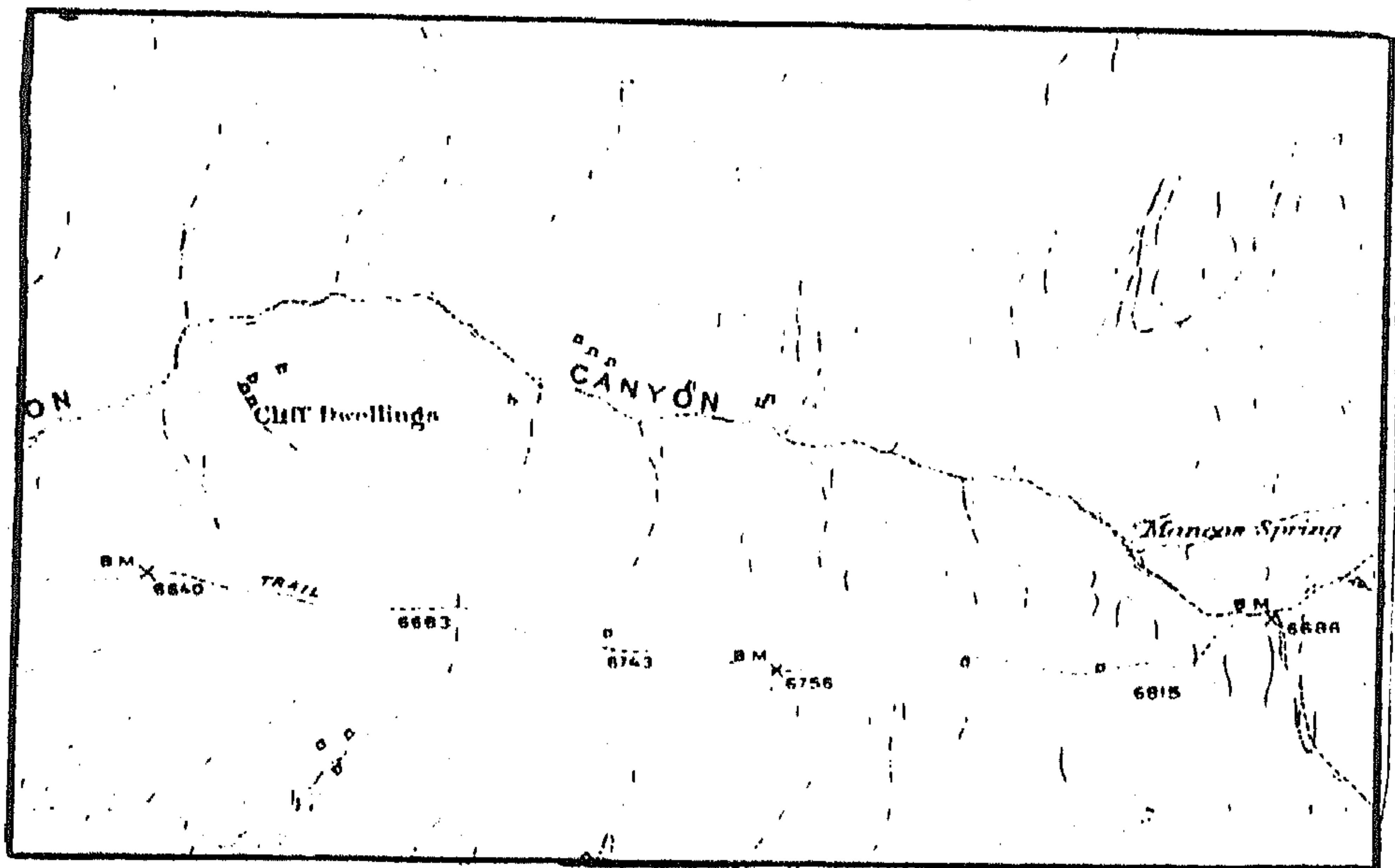
شكل رقم (٦٩) خانق سودا
