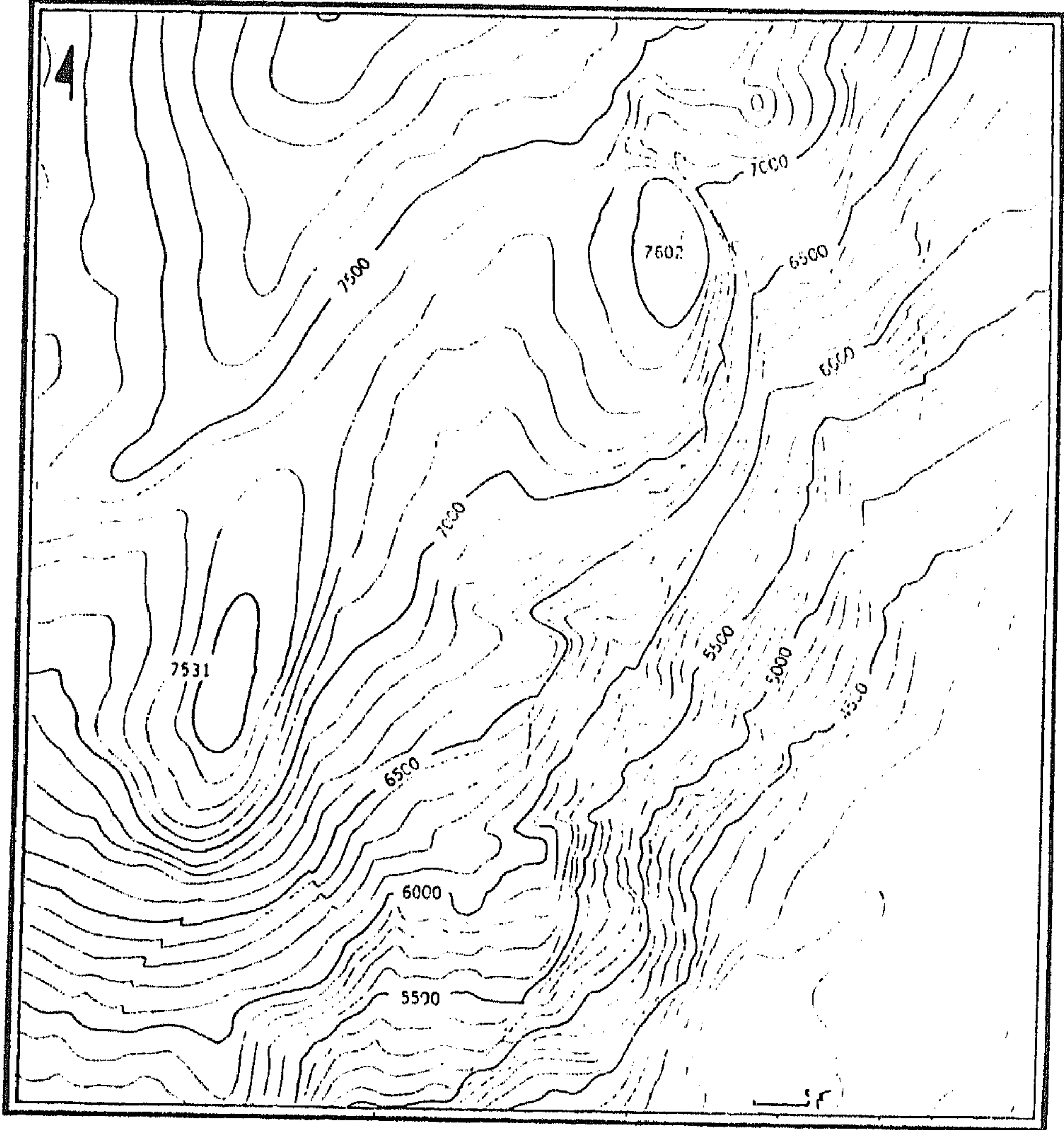
شكل رقم (١٣) الانحدار البسيط
