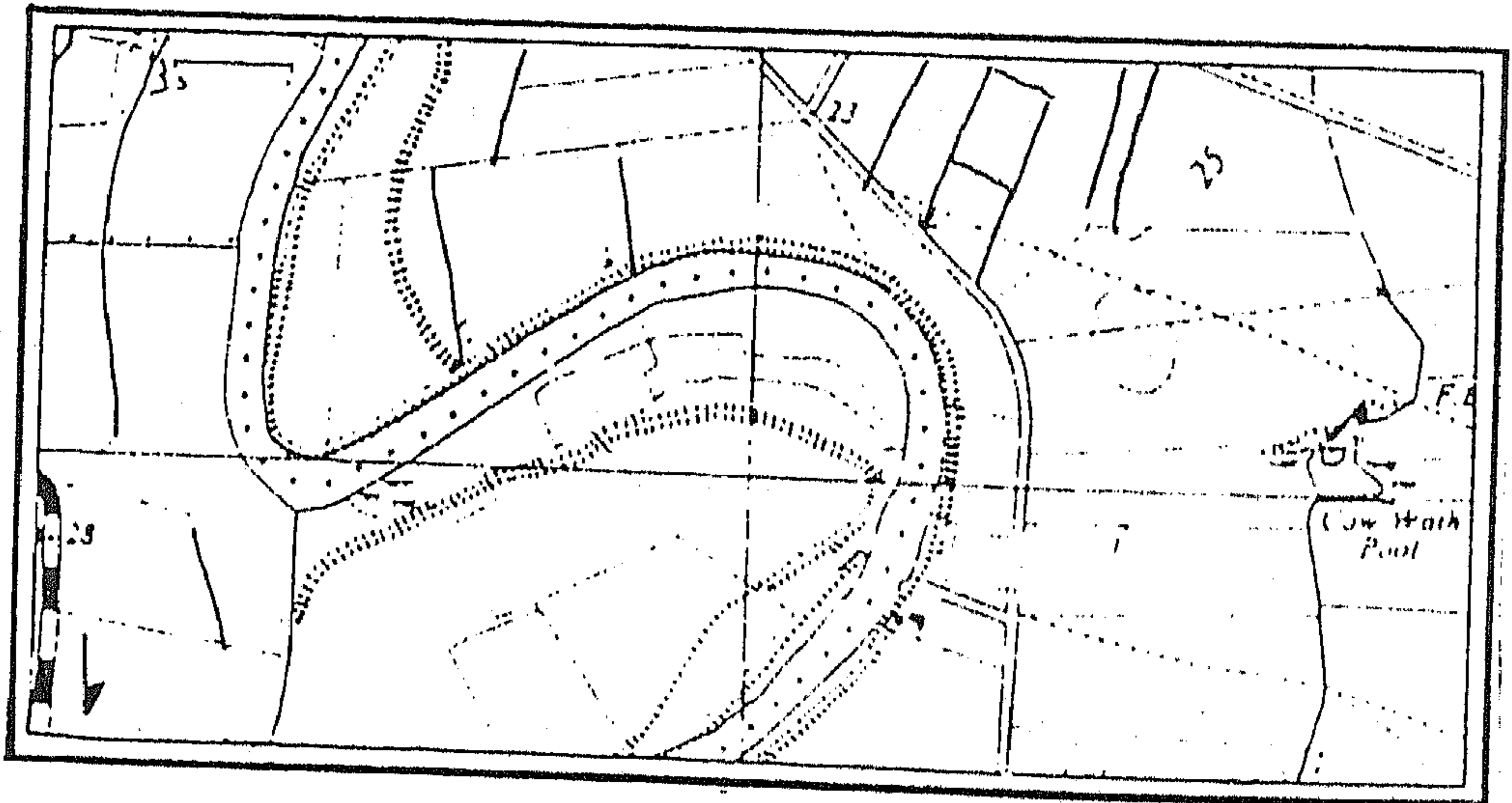
شكل رقم (٤١) ثنية نهر وسط سهل فيضى
