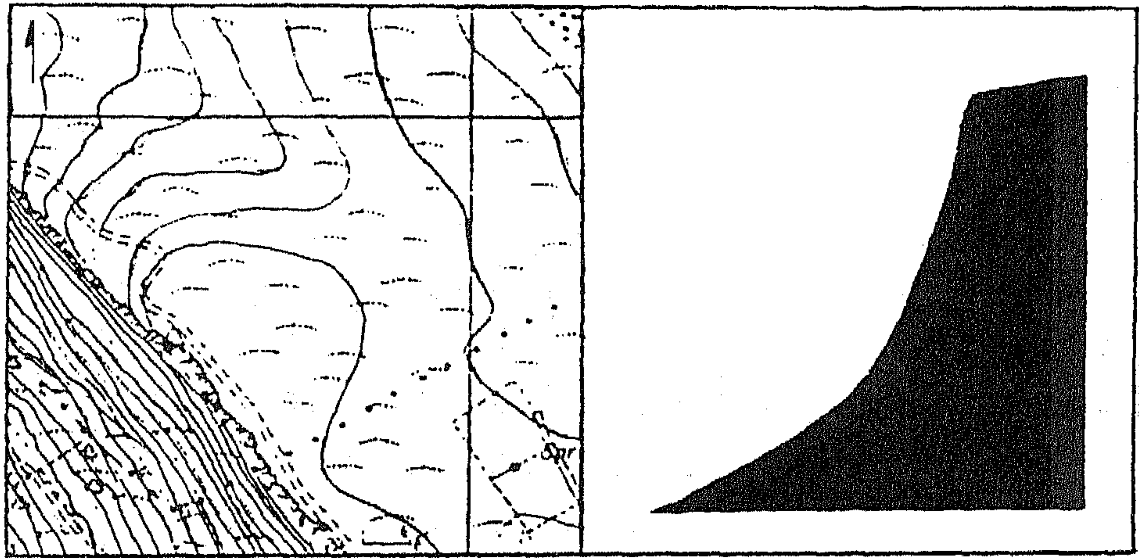
شكل رقم (٢٩) حافة حادة الانحدار بمنطقة دريشير
