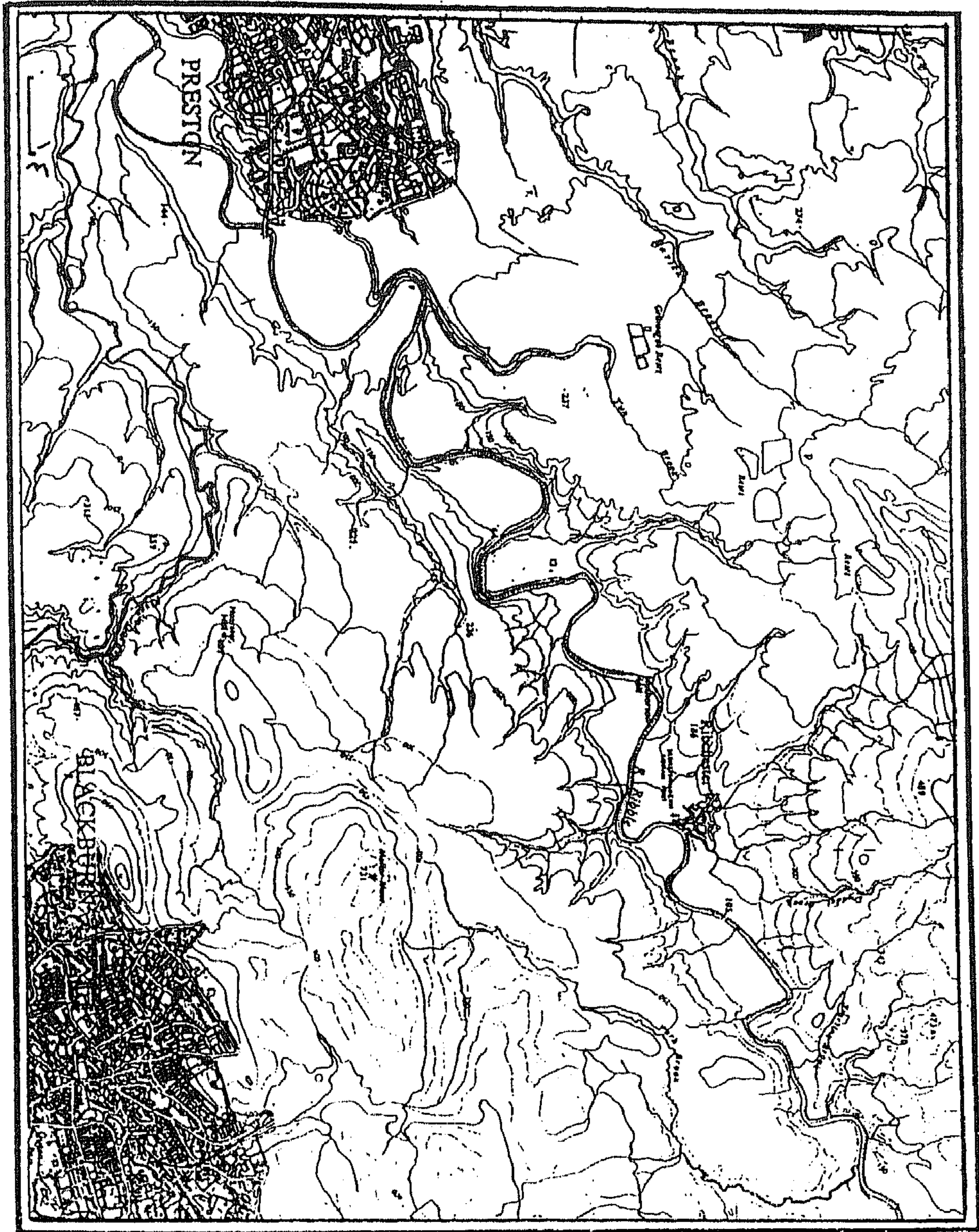
شكل رقم (٧٢) جزء من مجرى نهر ريبيل ببريطانيا
