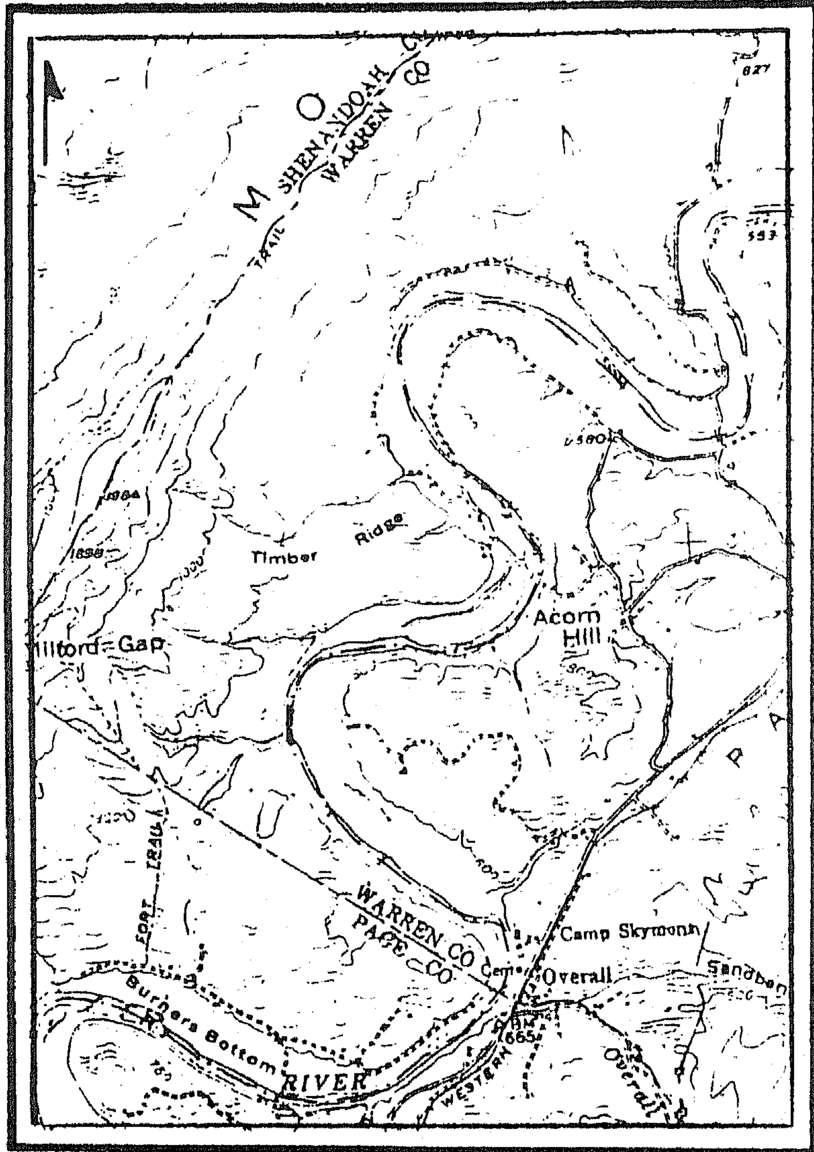
شكل رقم (٧١) نهر في مرحلة التضيق
