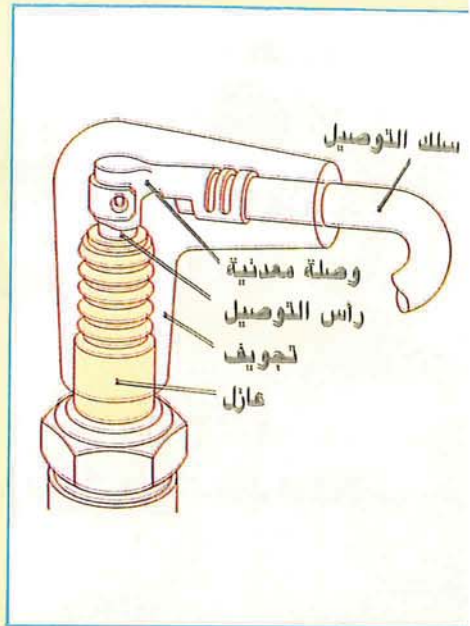
شكل (3) تفاصيل توصيل الكهرباء لشعلة الاحتراق :
