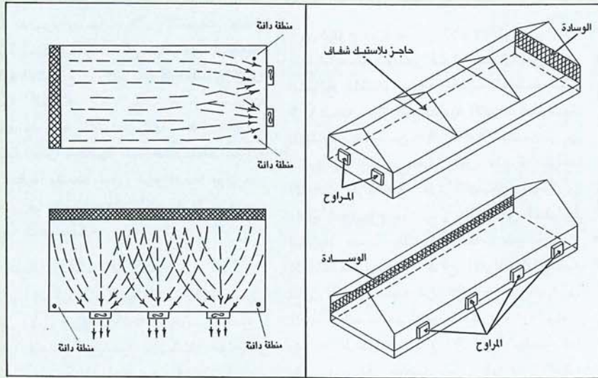
● شكل (٣ - ١) مواضع المراوح والوسائد والحواجز في البيت المحمي الجمالوني متناظر الانحدار . ● شكل (٣ - ب) مسارات الهواء داخل البيوت المفردة في الأوضاع المختلفة للوسائد والمراوح
