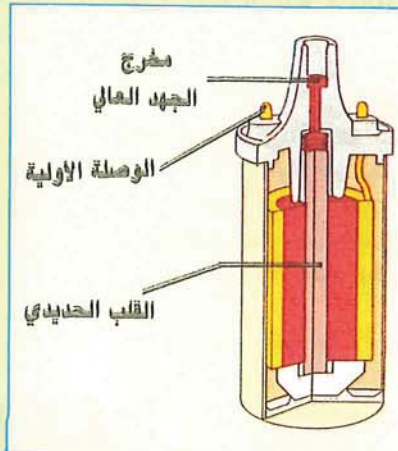
شكل (1) رفع الجهد في شكله الحقيقي
