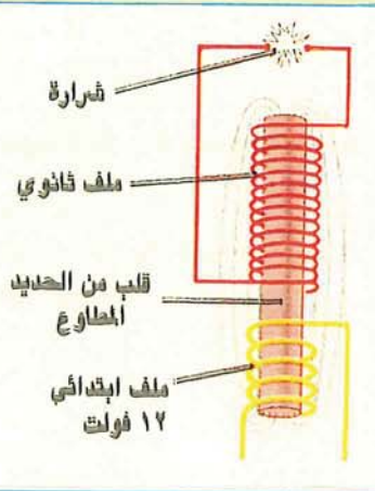
شكل (3) نظرية رفع الجهد
