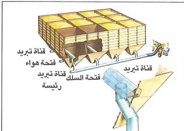
شكل (٦) طريقة تبريد الصوامع العادية .
