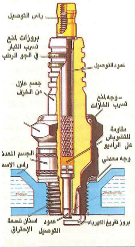
شكل (٢) شمعة الإحتراق
