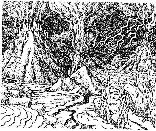
(شكل ٢-١) سطح الأرض منذ حوالي ٤ بليون سنة.
