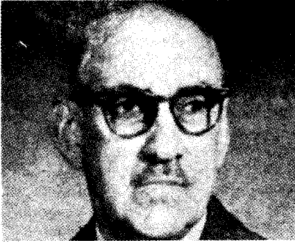
جای ویلسون آئن
