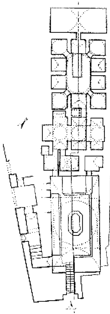
مسجد جامع قزوین - نقشه کتیبه ای - ۱۳۰۰ هجری قمری مقیاس ۱:۱۰۰
