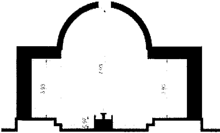
- شكل (١١٧) : قطاع داخلي في براني حمام العتيقة خارج باب قنسرين - حلب . عن : مديرية مدينة حلب القديمة - مركز التخطيط والدراسات م. ماجد زمار
