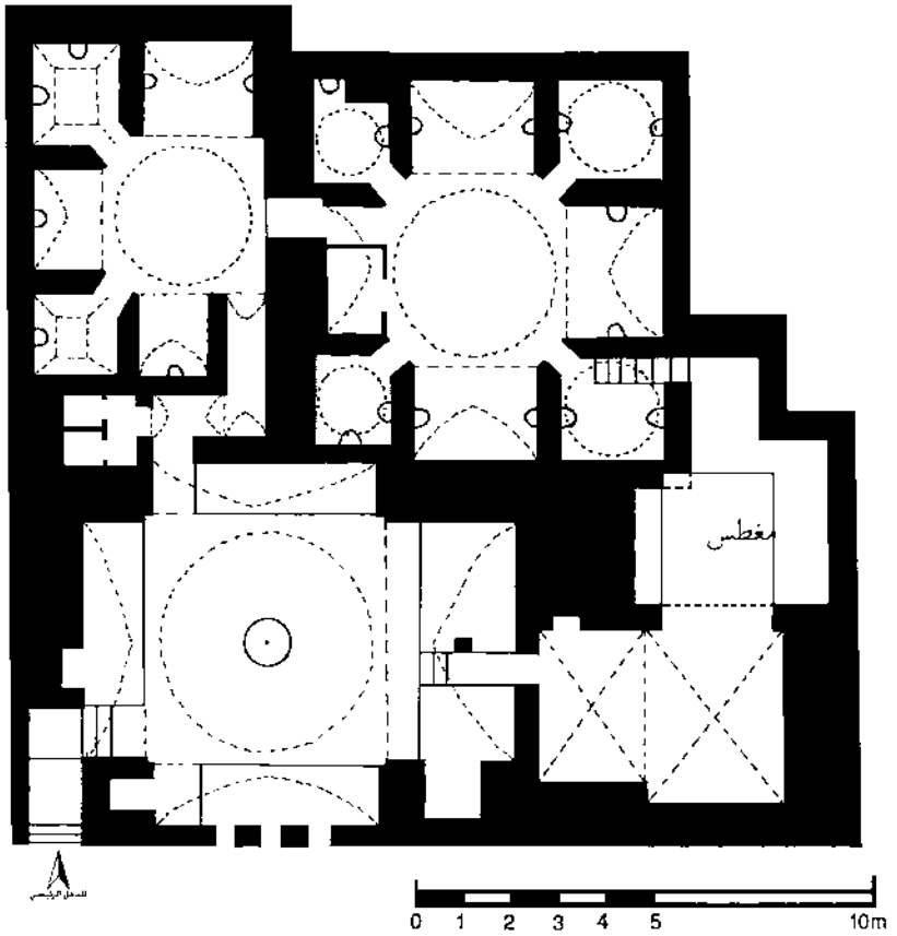
- شكل (67) : المسقط الأفقي لحمام الصالحية بشارع باب الخمام - حلب الوضع الراهن للحمام مقياس الرسم 100/1 عمل الباحث (بعد تصغيره)
