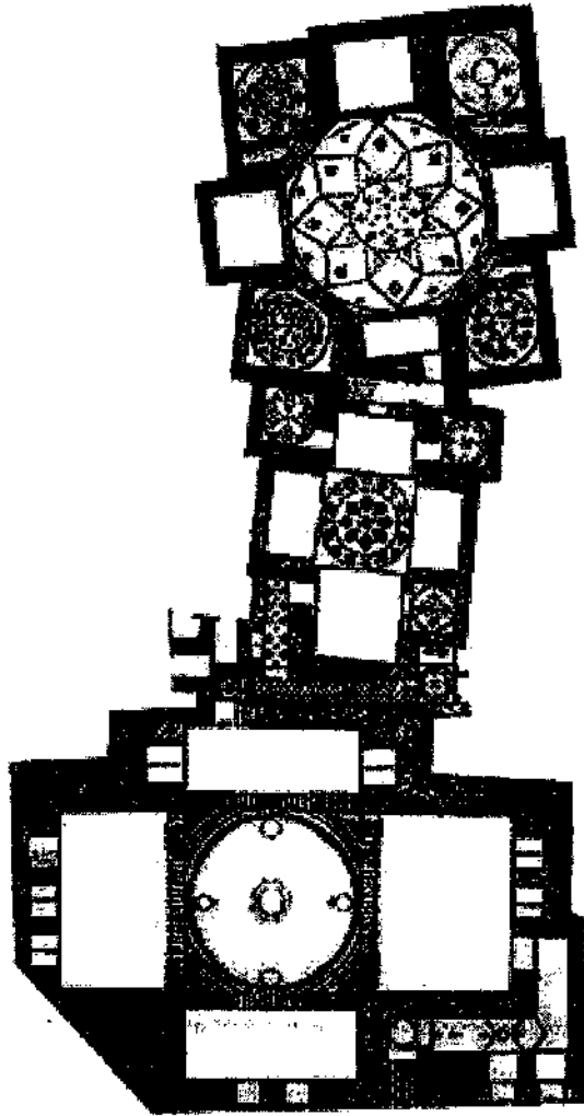
- شكل (50) : شكل يوضح أساليب توزيع القطعيات بأشكال زخرفية مختلفة على القباب والأقبية التي تغطي وحدات الحمام . عن : معمورة آثار حلب
