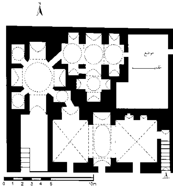
- شكل (2): المساحة الأفقية حمام بزاز - الوضع الراهن - عمل الباحث
