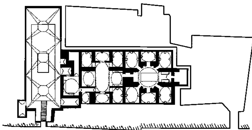
- شكل (4) : مسقط أفقي حمام النحاسين قبل الكشف عن الحمام الثاني عن : . . . Atef, P 142, Fig, 32 , ( J ) sauvaget
